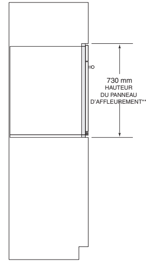
VUE LATÉRALE
