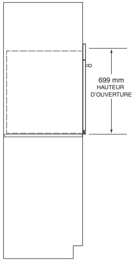
VUE LATÉRALE
