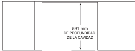
VISTA SUPERIOR
