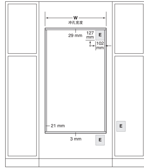
前视图
