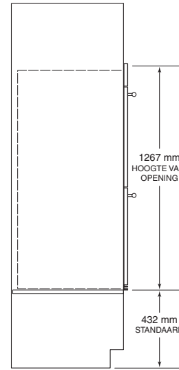
ZIJAANZICHT
