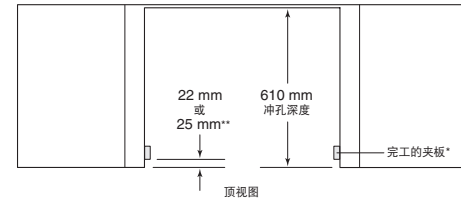
顶视图
