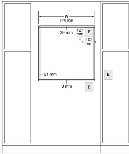
前视图
