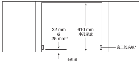
顶视图
