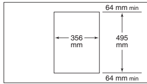
AUSCHNITT ARBEITSPLATTE
