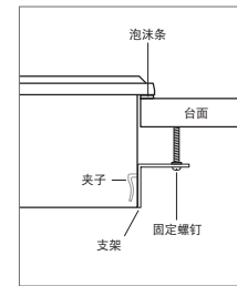
模块安装。
